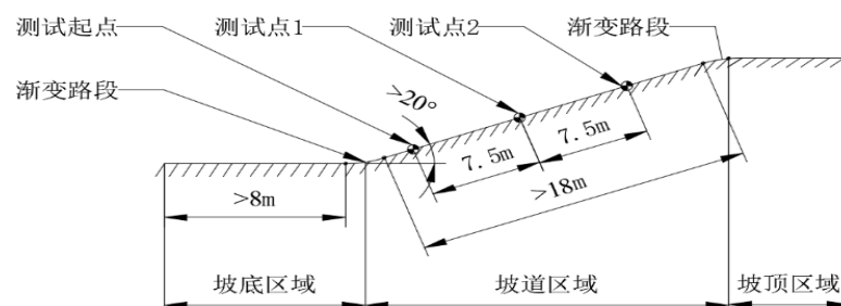
图A.1 试验坡道
